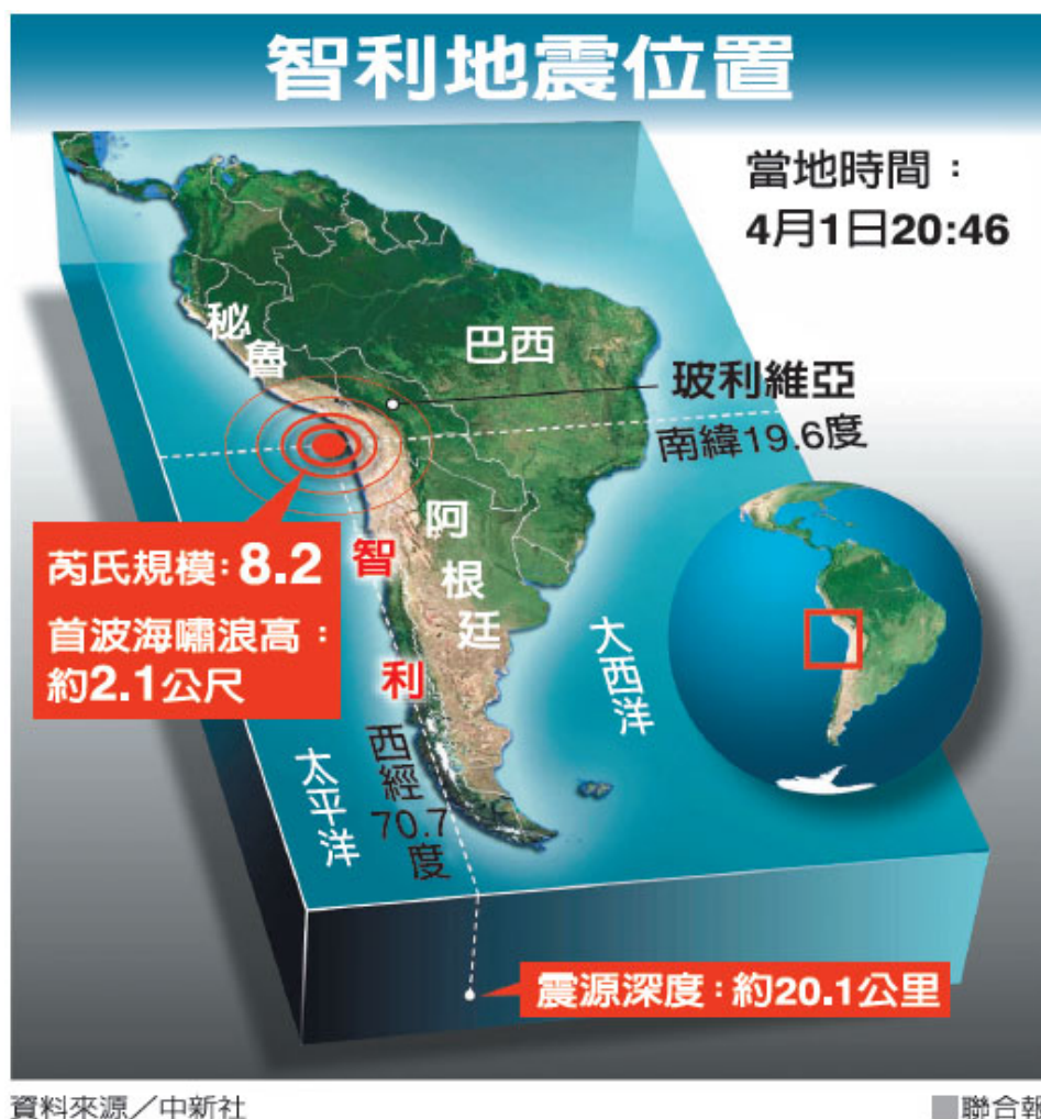
(圖 2. 智利地震圖)
